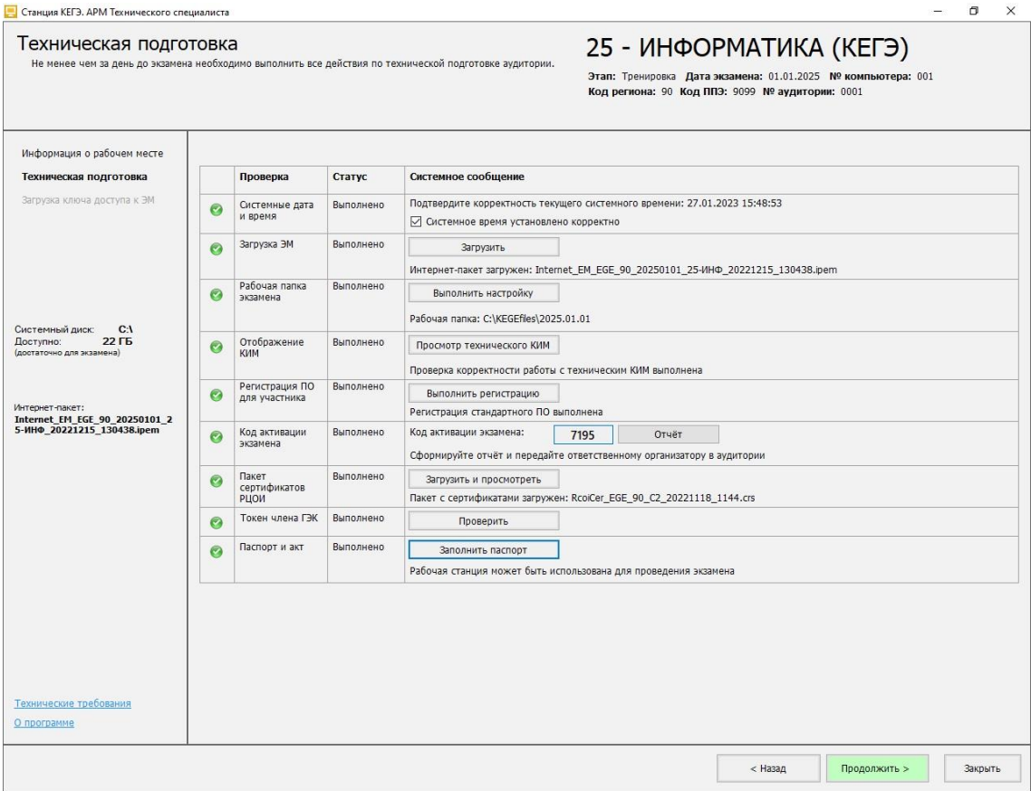
Рис. 6.42. Техническая подготовка и контроль готовности завершены
